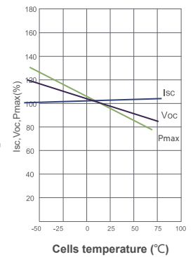
Isc, Voc, Pmax temperature
