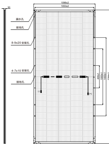
产品图示 单位: mm
