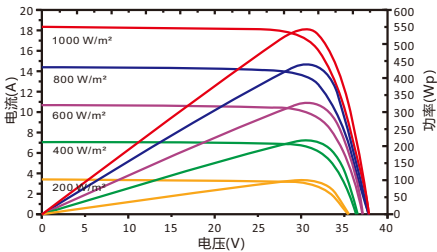
RSM110-8-545BMDG 不同辐照度下, I-V 曲线图
