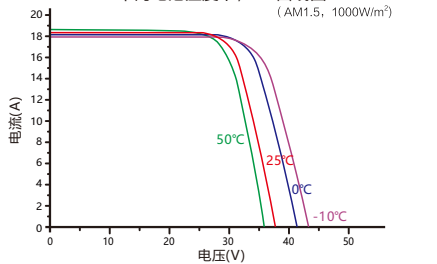
不同电池温度下, I-V 曲线图 (AM1.5, 1000W/m²)
